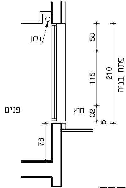
חיתך
