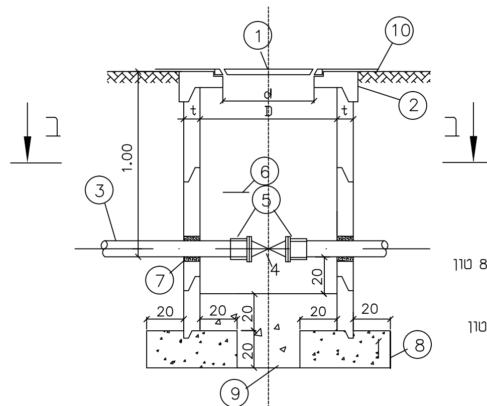
חתך א-א
