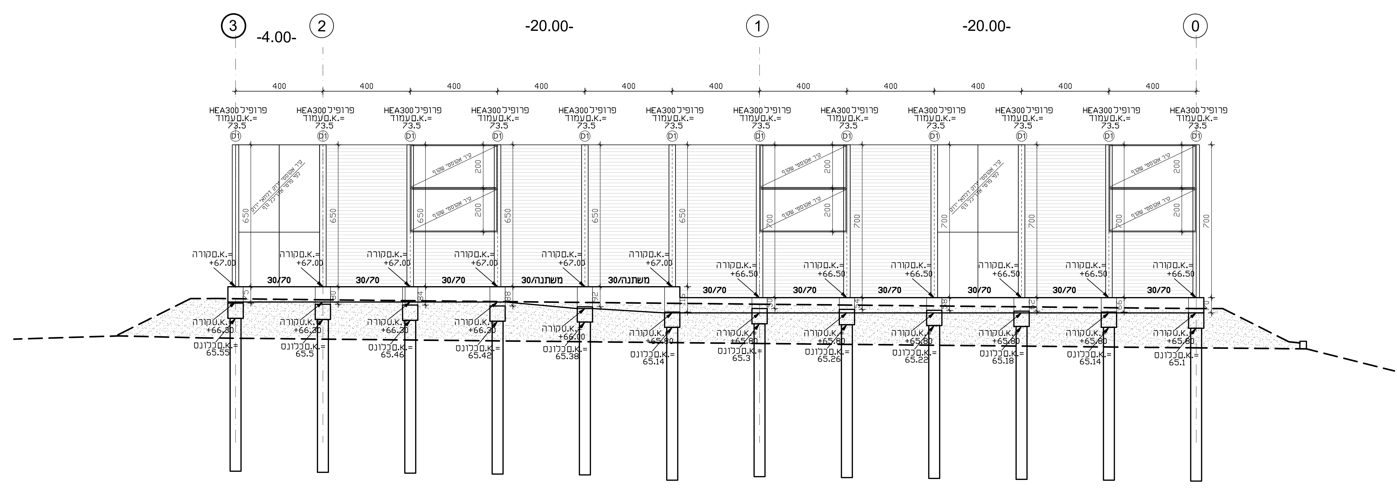
פרישת קיר א' חתכים 2-0
